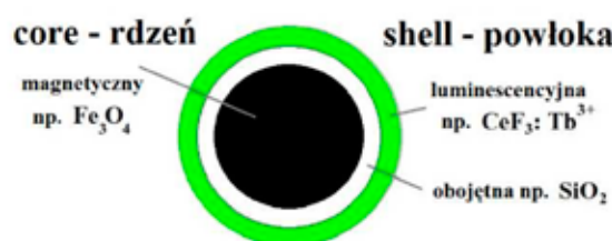
Rys. 2. Schemat budowy nanostruktur typu core/shell
