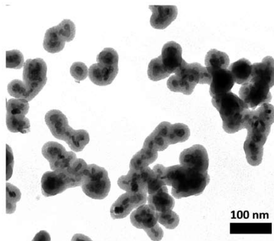
Rys. 5. Zdjęcie TEM modyfikowanych powierzchniowo nanocząstek typu core/shell – \text{CeF}_3:\text{Tb}^{3+}/\text{SiO}_2/\text{NH}_2
